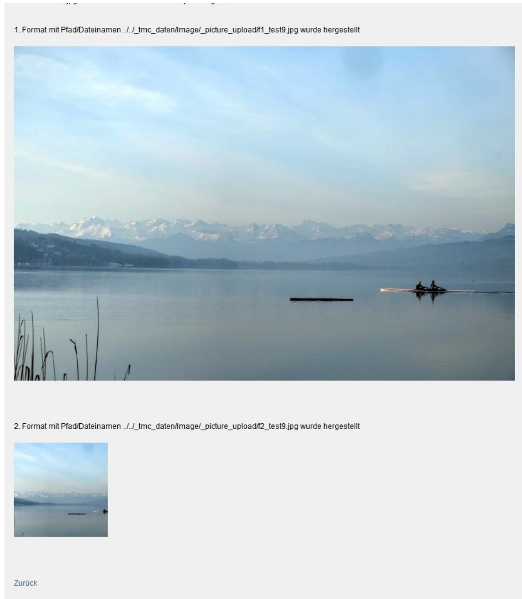
Bild3: Resultatseite
