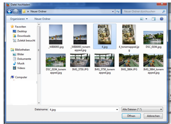
Bild2: Dateifenster
